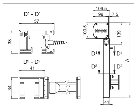
VD5100/1: Vägghäring utan clipssystem och monteringsfäste A = totalhöjd
