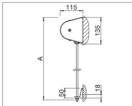
US3510/2 Väggmontering
