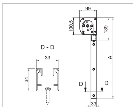
VD5100/2: Montering i dörrar/fönster med motor A = totalhöjd
