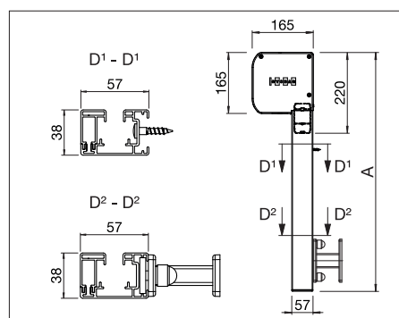
VS5600/1: Vägghäring med direktskruvförband och monteringsfäste A = totalhöjd
