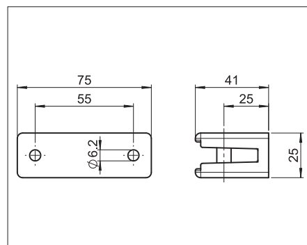
SR416 Upphängningsvinkel
