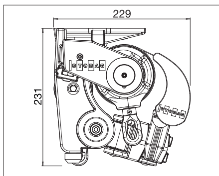
S8135 Takmontering
