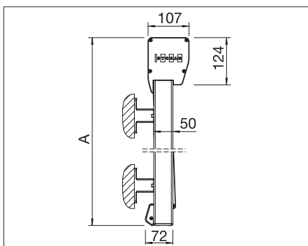
Med fyrkantig kassett, utfälld
