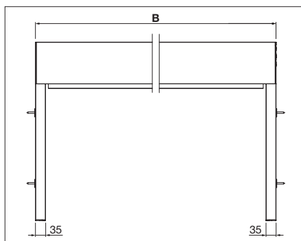
Monteringsplan för montage på väggen eller i dörrar/fönster
