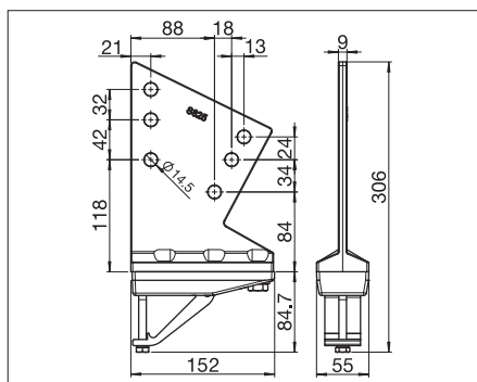
S825 Konsol för taksparrar
