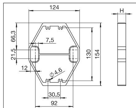
S821/1.. Underläggsplatta
