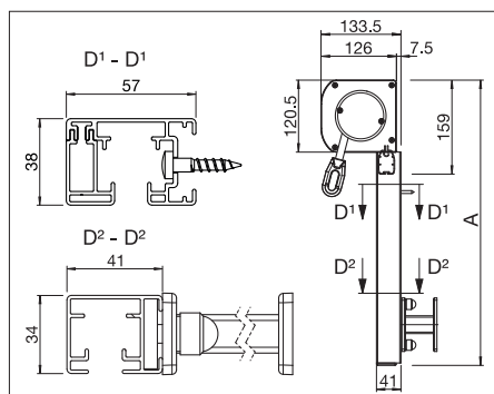
VS5200/1: Väggmontering utan clipssystem och monteringsfäste A = totalhöjd
