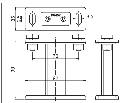
PS452/1 Monteringsfäste
