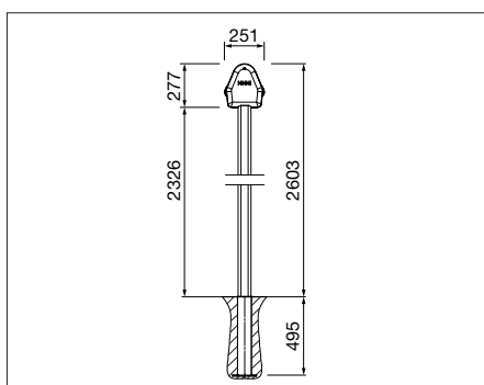
2-bensversion OS416/2 med markhylsa OS315
