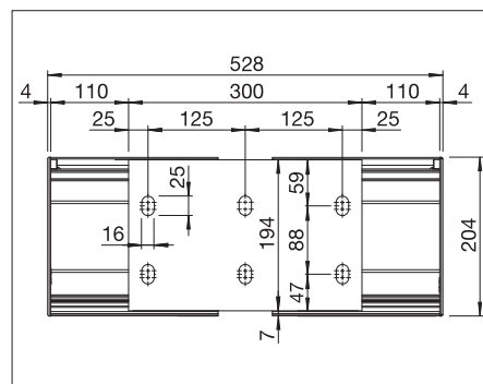
B423/2 Konsolfäste 300 mm
