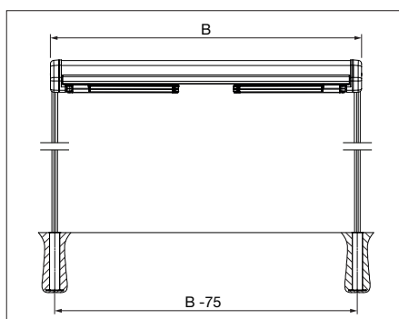
Version OS416/2 med markhylsa
