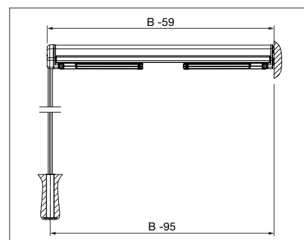
Version OS416/2 med markhylsa och väggfäste OS4010/1
