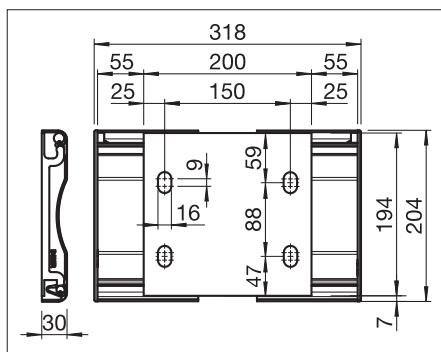
B423/1 Konsolfäste 200 mm
