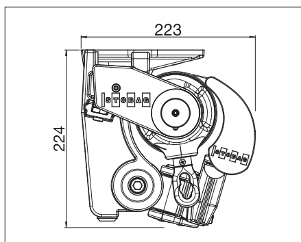
S8130 Takmontering
