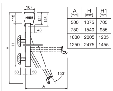
Vägghmontering med fyrkantig kassett
