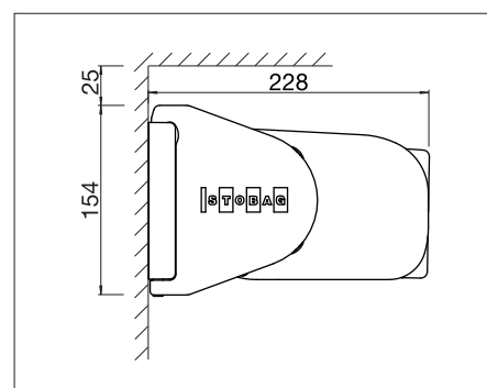
Väggmontering med fyrkantig utfällningsprofil
