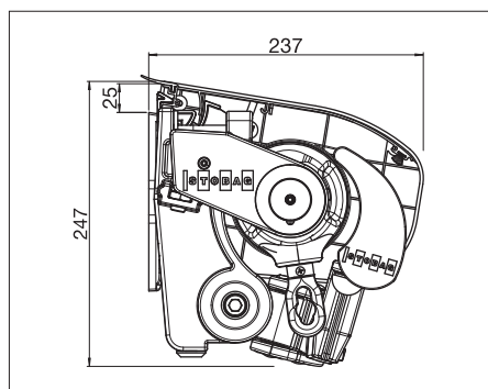
S8130 Väggmontering med skyddstak S877/2 och utfällningsprofil S894
