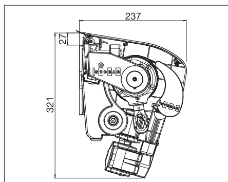
S8133 Väggmontering med skyddstak
