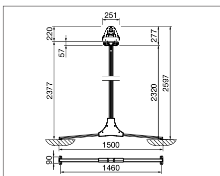
2-bensversion OS416/1 med tvärgående stödfötter OS412
