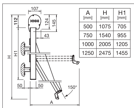
Vägghmontering med rundad kassett
