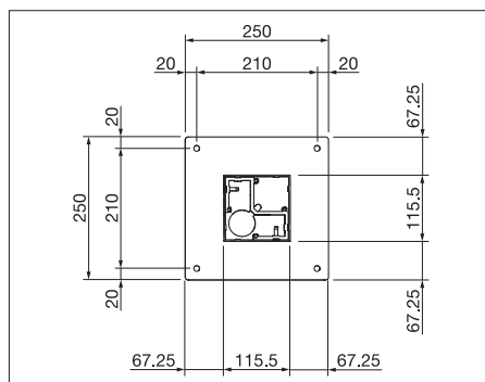
Tvårsnitt fotplatta TP313 (standard)
