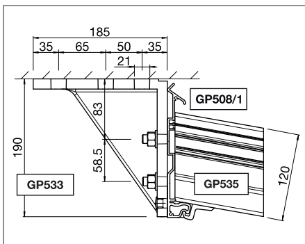
Takmontering
