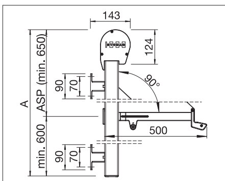
Med rund kassett, utfälld
