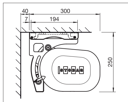
Takmontering
