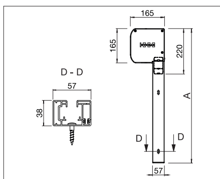
VS5600/2: Montering i dörrar/fönster med direktskruvförband A = totalhöjd
