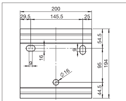
S563/1 Konsolprofil L = 200
