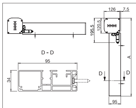
Väggmontering utan clipssystem A = totalhöjd
