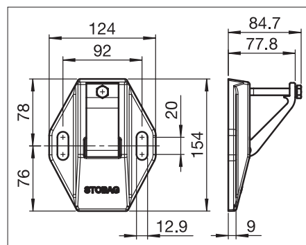
S821/1 Vägg-/takkonsol
