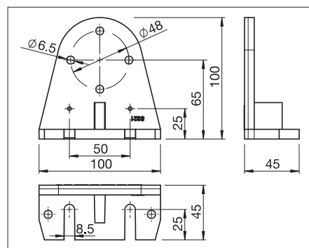
S321 Lagerskål
