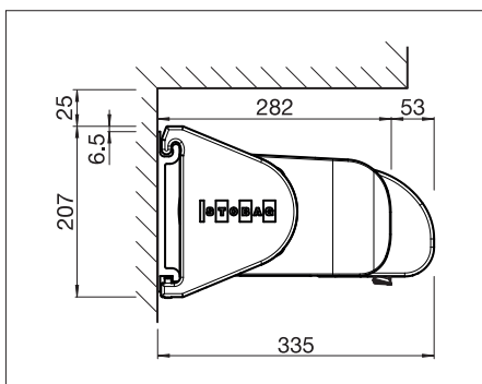
Väggmontering med AV Rundad utfällningsprofil
