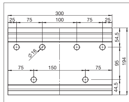
S563/2 Konsolprofil L = 300
