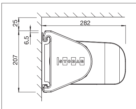
Väggmontering Rundad utfällningsprofil
