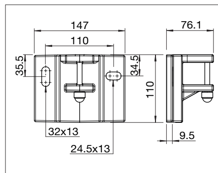
S221/3-1 Väggkonsol
