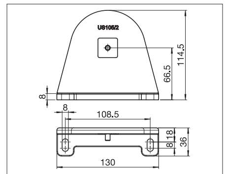
US105/2 Inställningskäpa
