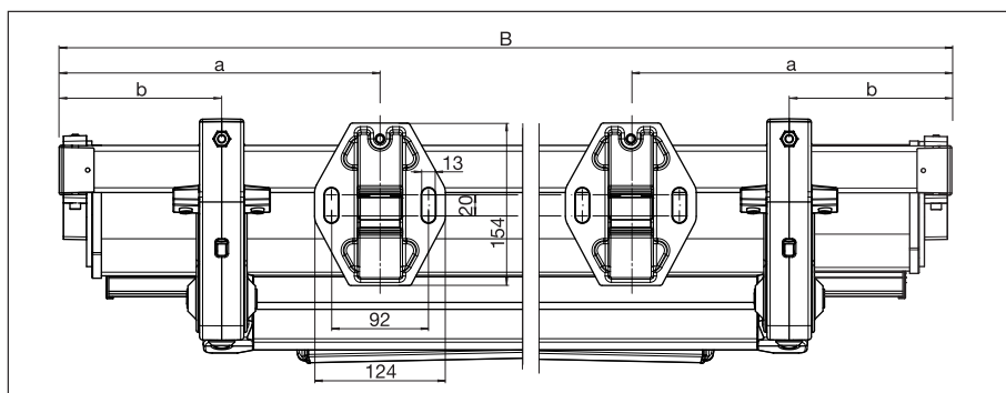
S8250 Monteringsplan B = totalbredd
