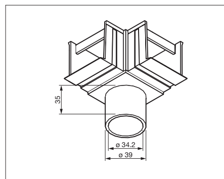
Standard-vattenränna WS
