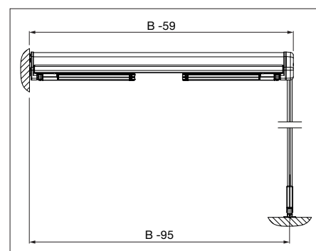
Version OS416/1 med tvärgående stödfötter och väggfäste OS4010/1
