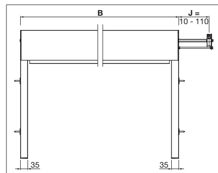
Monteringsplan med markisväxel
