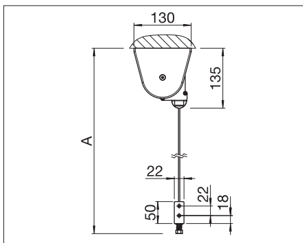
US3510/1 Täkmontering
