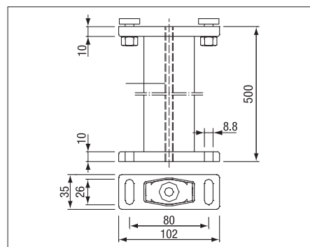
PS547 Monteringsfäste
