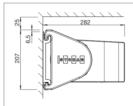
Väggmontering Fyrkantig utfällningsprofil
