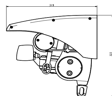
FA42 PC TAK
